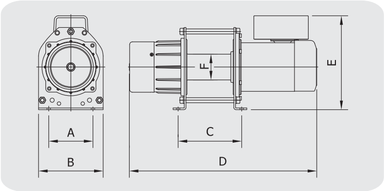
DIMENSIONS
