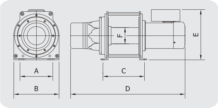
DIMENSIONS
