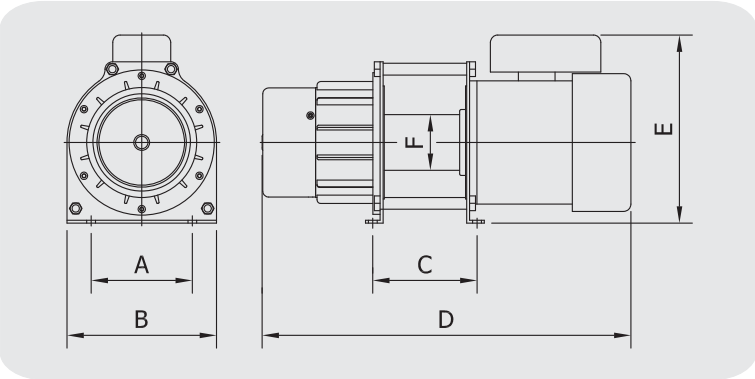
DIMENSIONS
